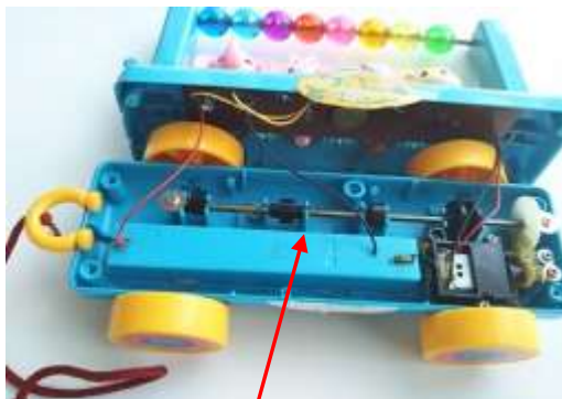
カムギア
